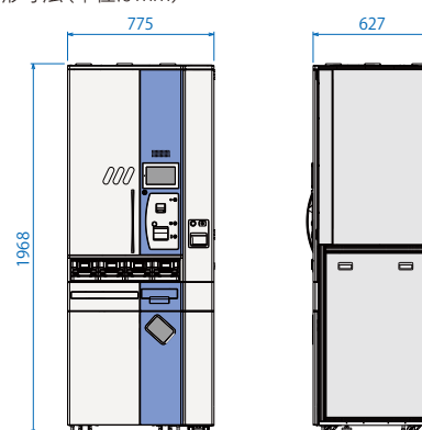
■外形寸法(単位はmm)
